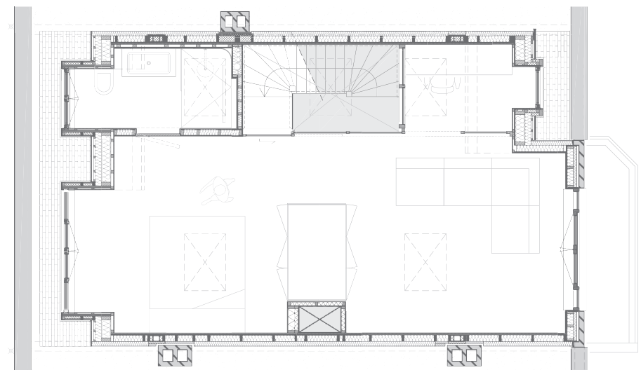
plattegrond en doorsnede
